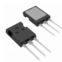
IXGX320N60A3 IXYS IGBT 600V 320A 1000W PLUS247
