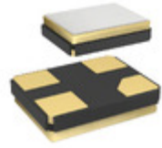
F216R-27.000 Fox Electronics OSC XO 27.000MHZ HCMOS SMD
